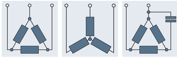
Соединение «треугольником»
